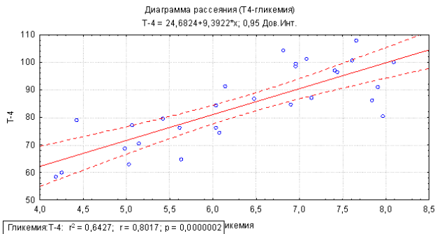
Рисунок 1 – Диаграмма рассеяния наблюдений в координатах исследуемых переменных (тироксин – гликемия) при анализе корреляционной связи в условиях острой алкогольной интоксикации
