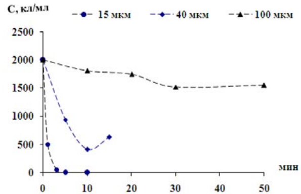
График 2 - Зависимость концентрации бактериальных клеток в фильтрате от времени при использовании фильтров с разным диаметром пор (диаметр пор = 15, 40 и 100 мкм, E = 9,4 В/см, скорость фильтрации – 10 мл/мин)
