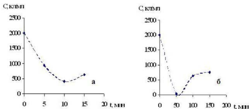
График 3 (а, б) - Зависимость изменения концентрации бактериальных клеток E.coli в фильтрате от времени при различных скоростях электрофльтрации ( d_{пор} = 40 мкм, E = 9,4 В/см, а) V = 10 мл/мин, б) V = 1 мл/мин)
