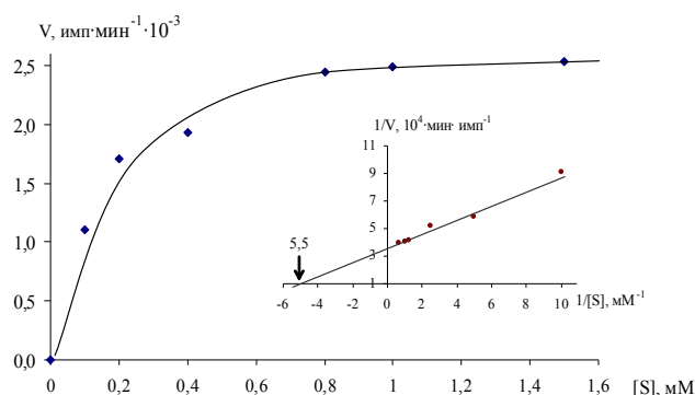
Рисунок 3 – Зависимость начальной скорости (ФРПФ) реакции от концентрации Р-5-Ф
